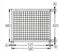
ホットボックス金網8段 ホットボックスの棚に挿入する 金網の寸法
